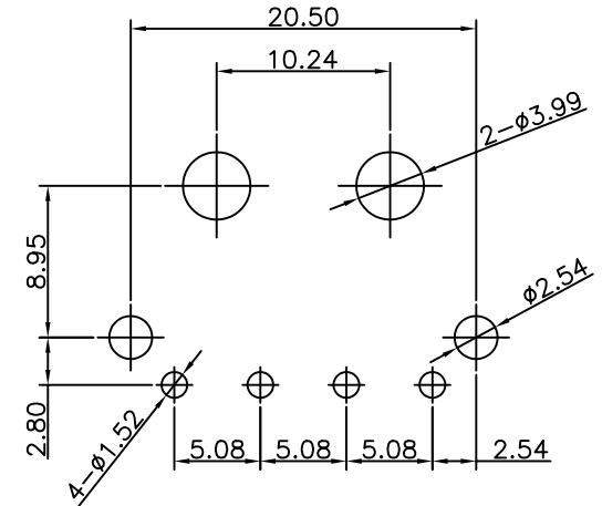
P.C.B LAYOUT
